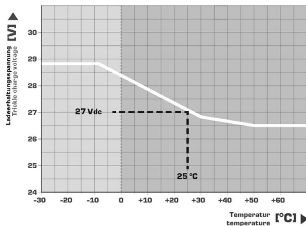
Abbildung 8: Kompensationsladekennlinie
