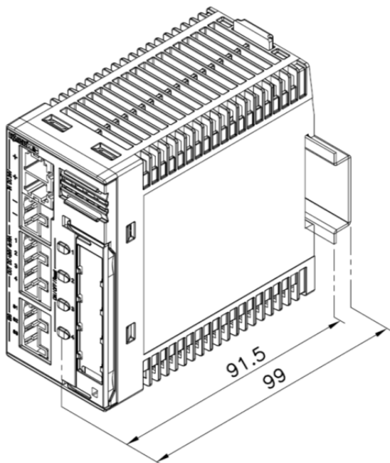
Abmessungen 4/2-Kanal-Module mit steckbarer Anschluss-technik
