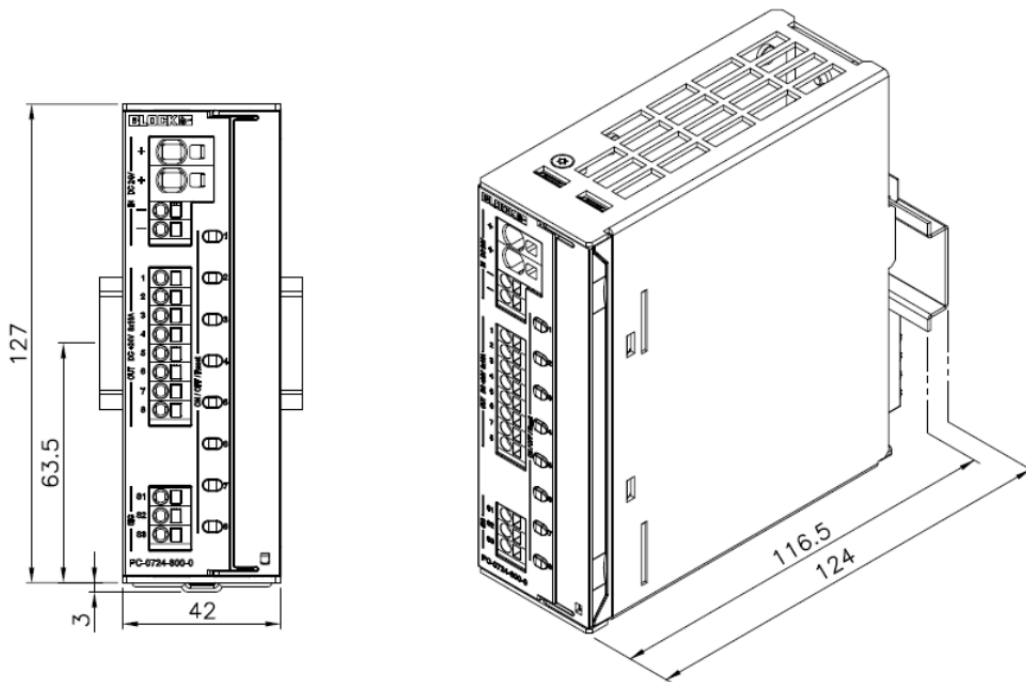
Abmessungen 8-Kanal-Module
