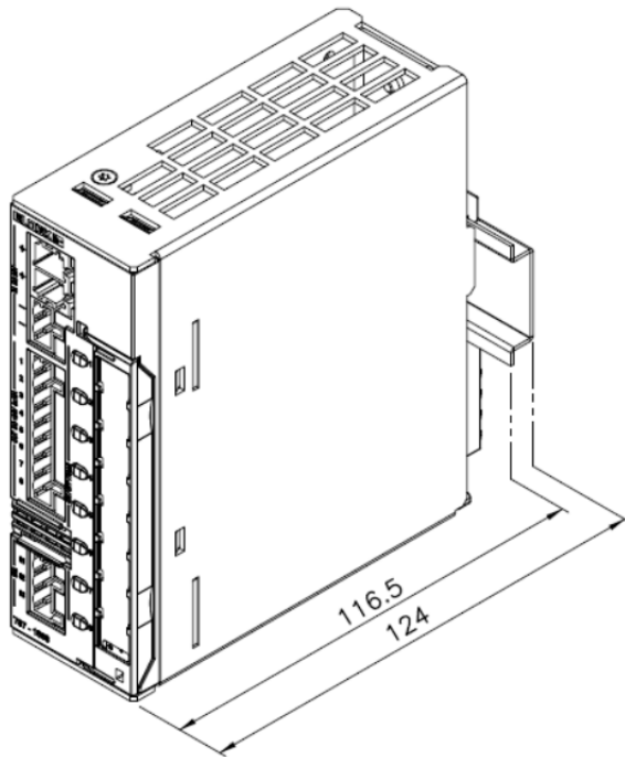
Abmessungen 4-Kanal-Module mit steckbarer Anschluss-technik
