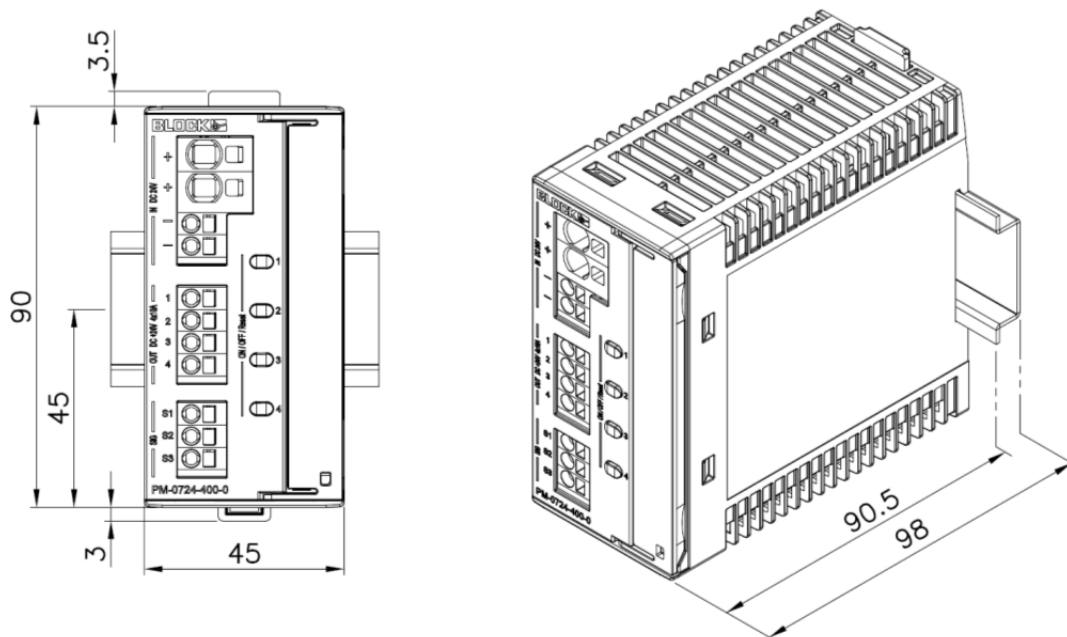
Abmessungen 4/2-Kanal-Module
