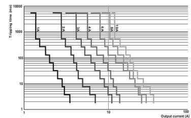
Fig. 3 Auslöseverhalten der Schutzschalter Tripping characteristics of the circuit breakers
